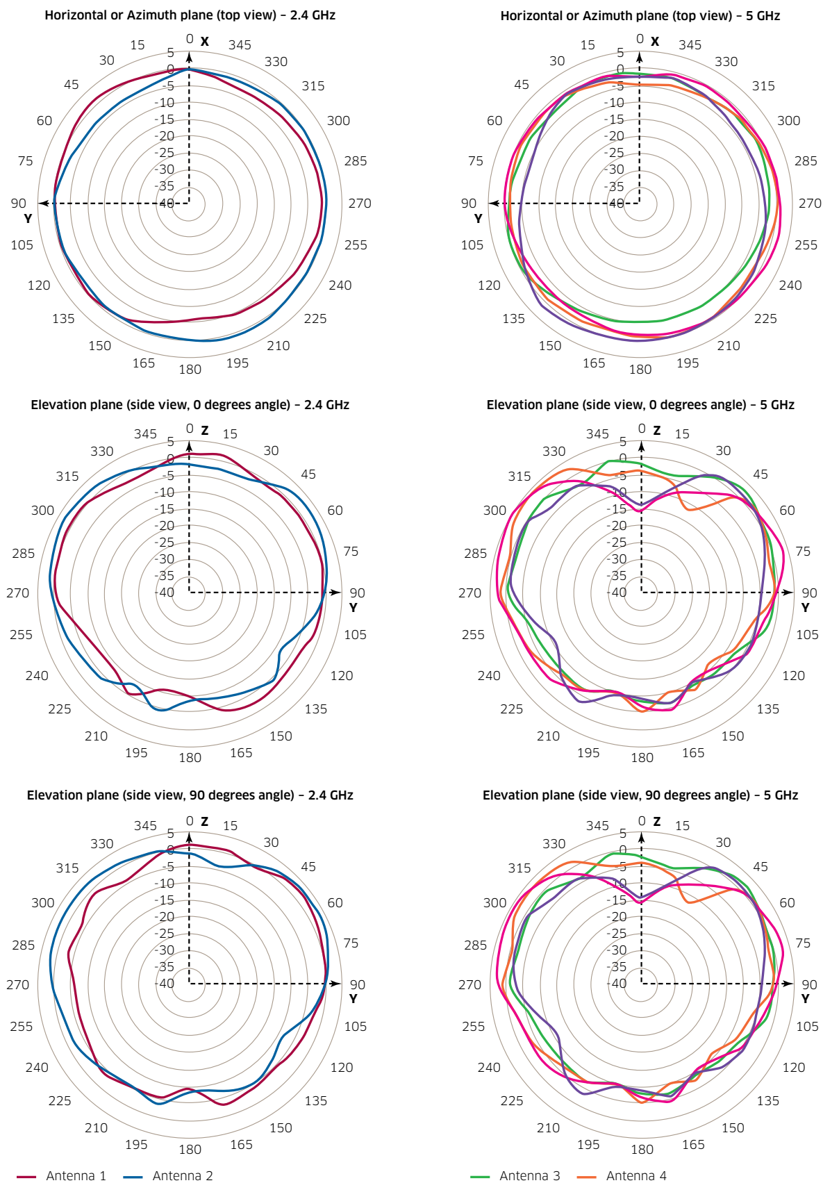
Figure 1. Diagramme de rayonnement OmniAccess Stellar AP1221
